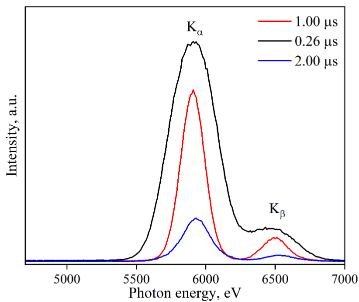
รูปที่ 3 เปรียบเทียบ XRF ของสารมาตรฐานโลหะ Mn ระหว่าง peaking time ที่ 0.26 1.00 และ 2.00 \mu s
