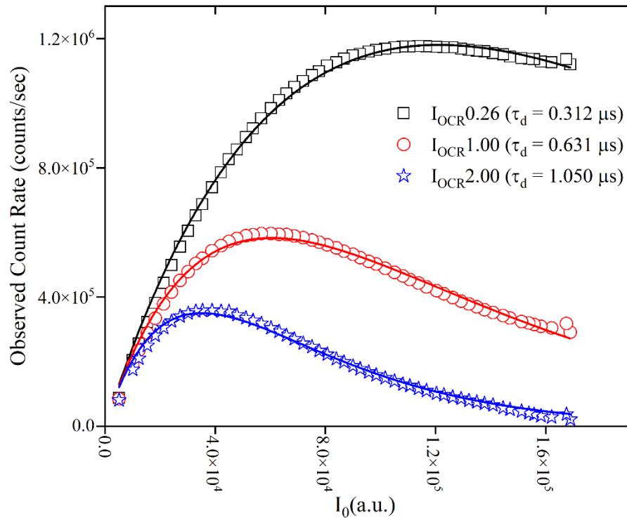
รูปที่ 4 ความสัมพันธ์ระหว่าง OCR และ I_0 สำหรับ Peaking Time 0.26, 1.00 และ 2.00 \mu s พร้อมเส้นฟิตด้วยแบบจำลอง Paralyzable เพื่อหาค่า P และ \tau_d ของระบบ
