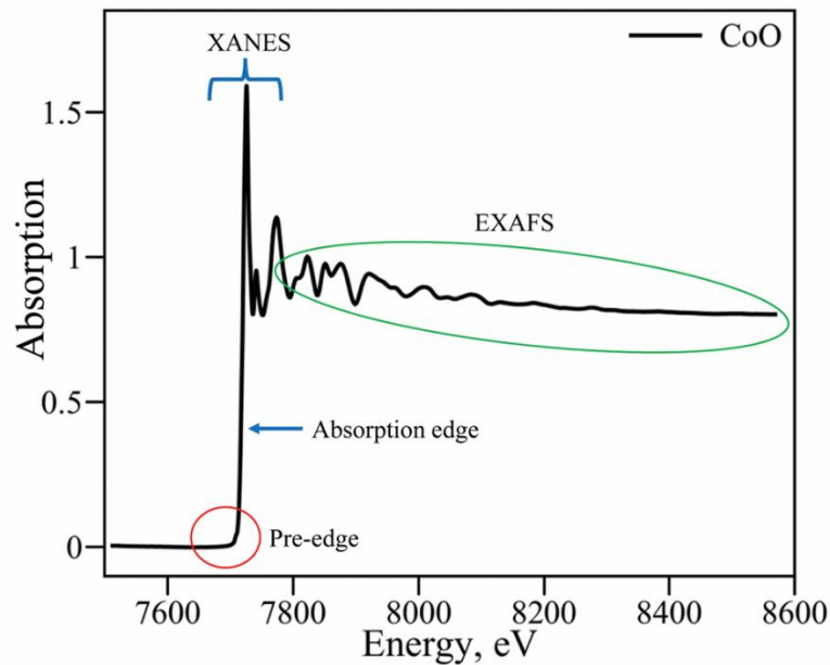
รูปที่ 1 ตัวอย่างสเปกตรัม XAS
