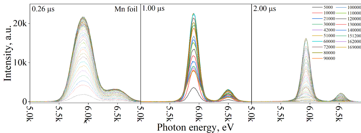
รูปที่ 2 สเปกตรัม XRF ของโลหะ Mn ที่ตรวจวัดด้วย SDD สำหรับค่า Peaking Time ต่างกัน (0.26, 1.00 และ 2.00 \mu s)
