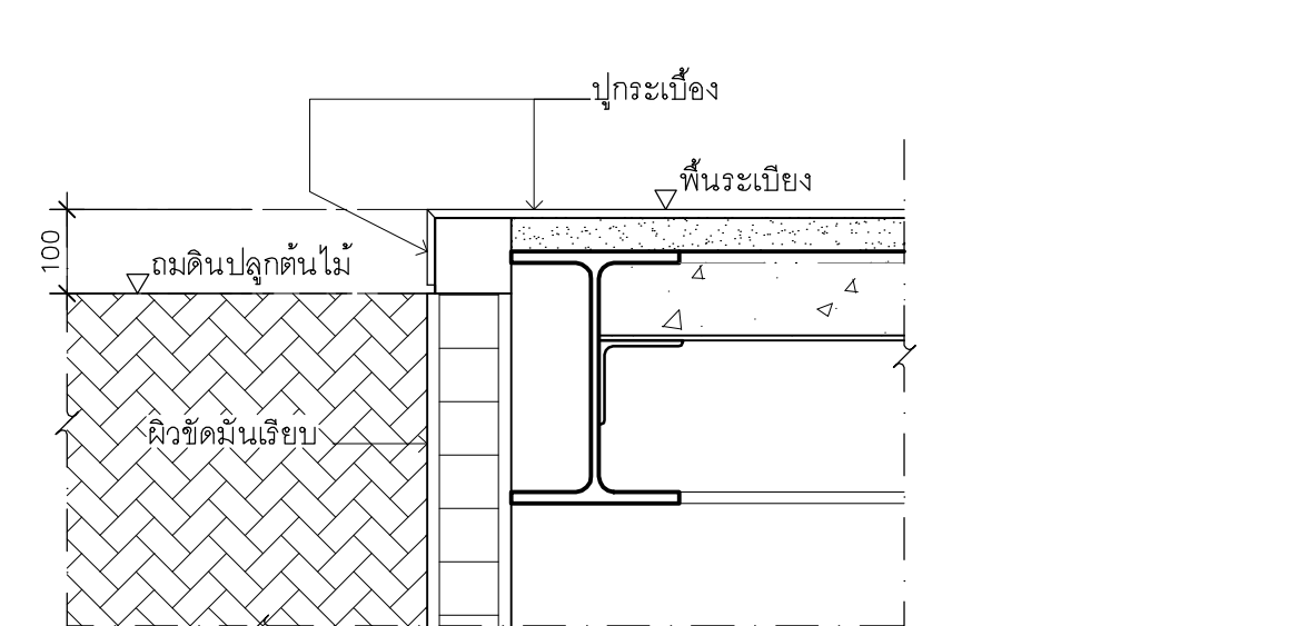
แบบขยาย
