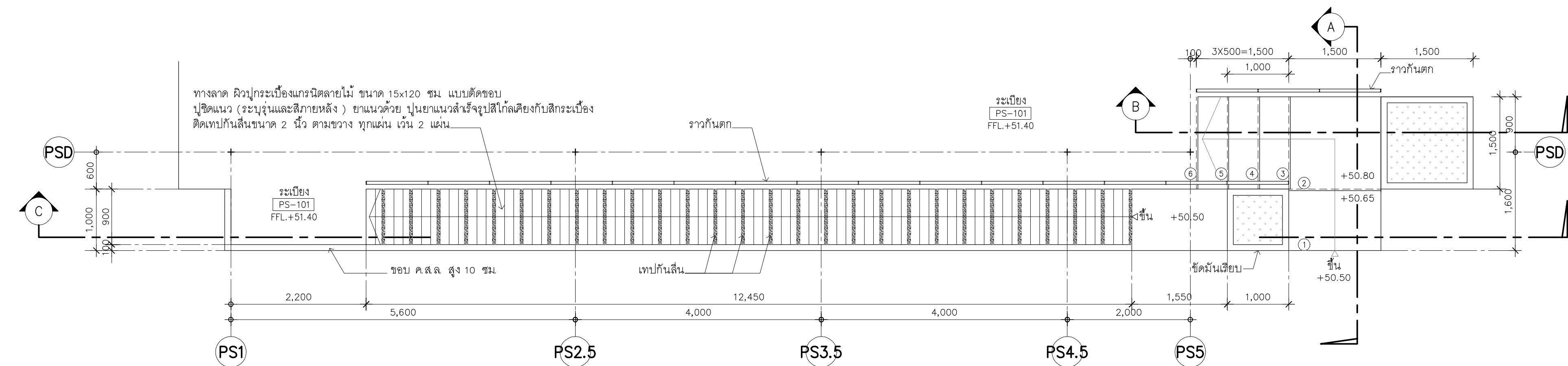
แปลนขยายบันได ST-01,RD-01
