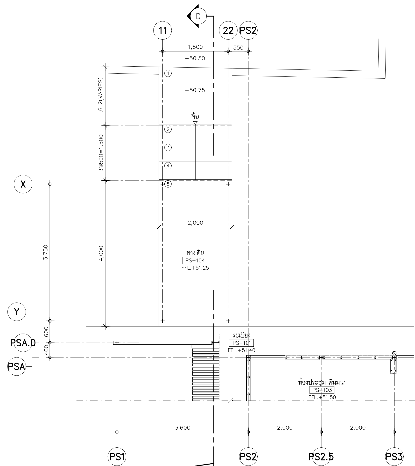
แปลนขยายบันได ST-02
