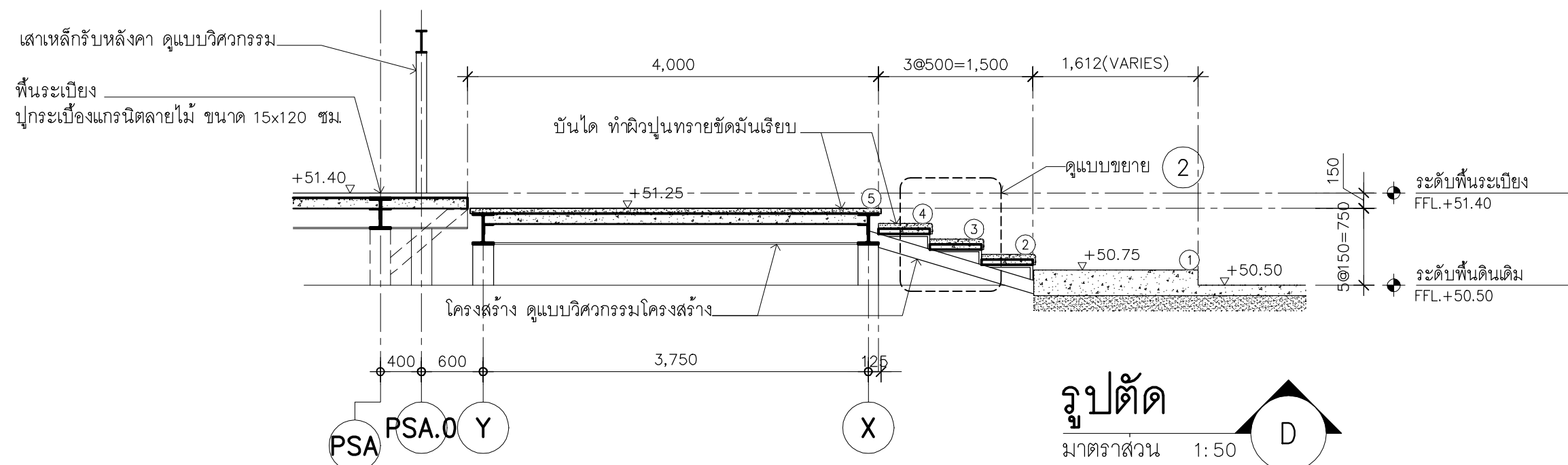
รูปตัด
